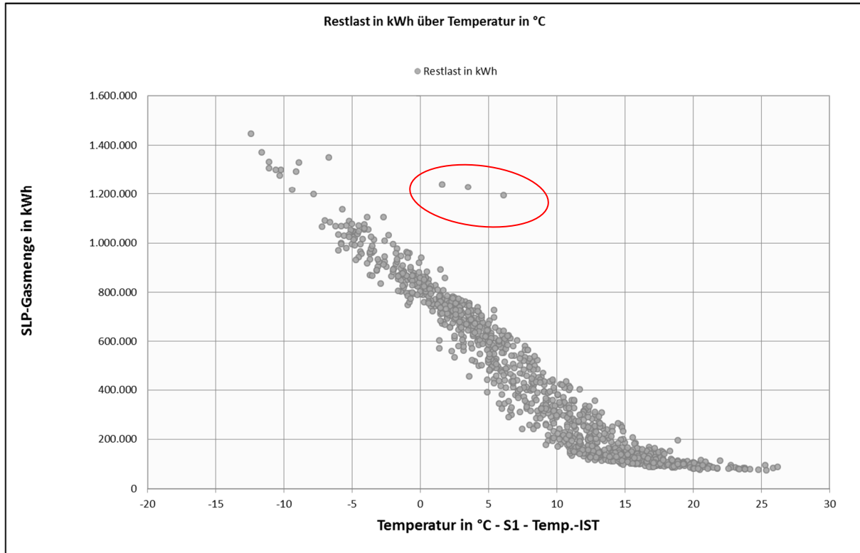
Abbildung 28 Restlastpunktewolke in Abhängigkeit zu der Tagesmitteltemperatur mit Datenfehler
