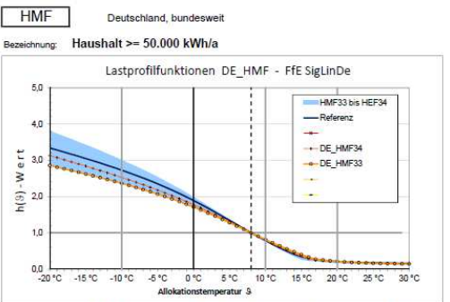
Profilkoeffizienten FfE SigLinDe
